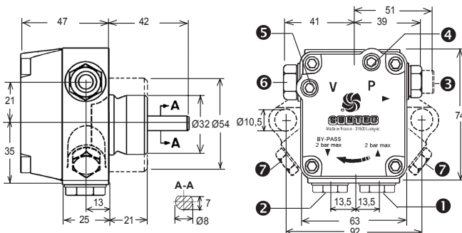
Насосы модификаций 4,6
