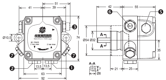
Насосы модификации 2
